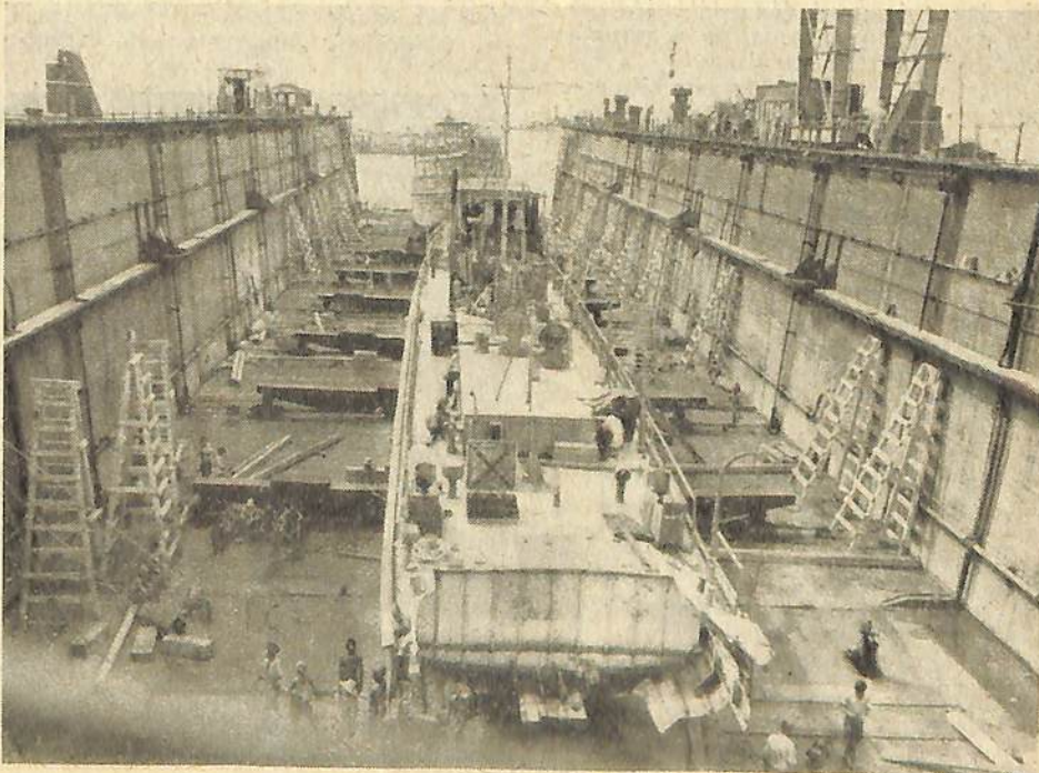
Batavia herleeft. Herstelwerkzaamheden aan het droogdok te Tg. Priok.
